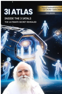
3i Atlas
